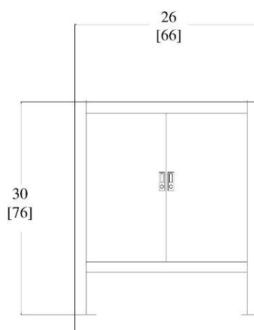
Az állvány elhelyezése és az ajánlott helyszükséglet Ábra 2.0
