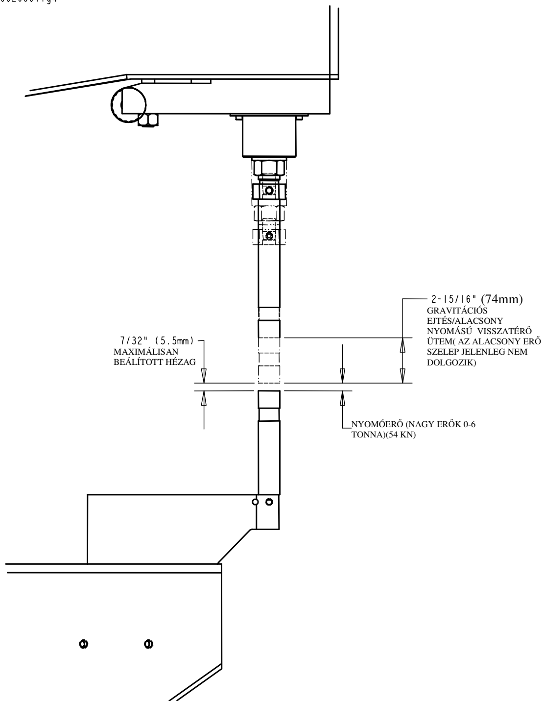
LÖKETHOSSZ ÁBRA 4.0
