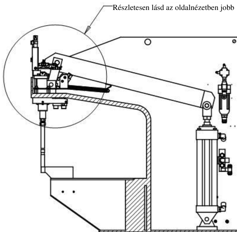
Présgép szerkezeti felépítése Ábra 3.2-2
