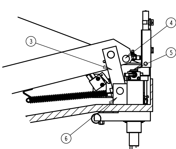
Préskulissza oldalnézetben
