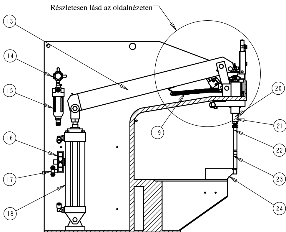
Présgép szerkezeti felépítése Ábra 3.2-1
