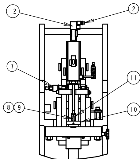
Préskulissza előlnézetben
