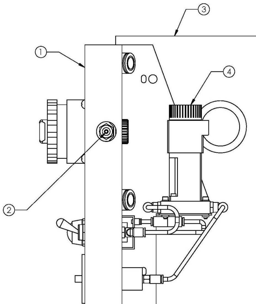
AZ IDŐZÍTŐ/VEZÉRLŐ DOBOZ ELTÁVOLÍTVÁ/ ÁBRA 3.4
